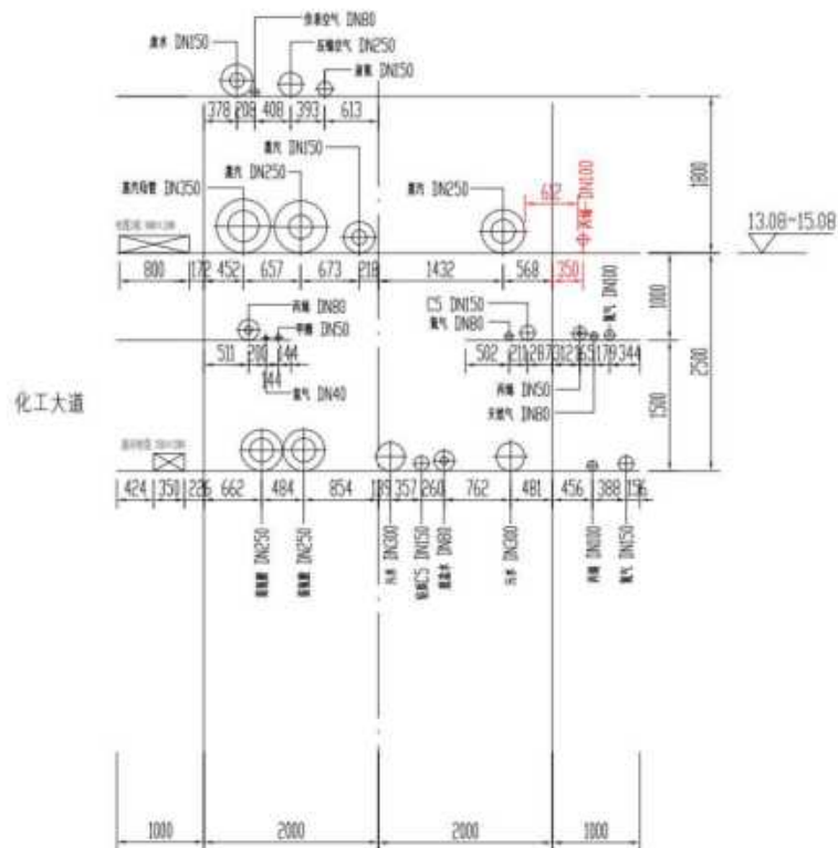
图 2-2 (a) 柱 9301~9334 段
